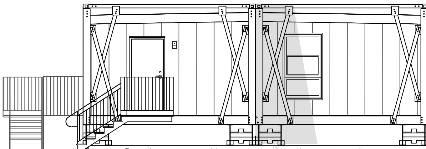
ÉLÉVATION ARRIÈRE
