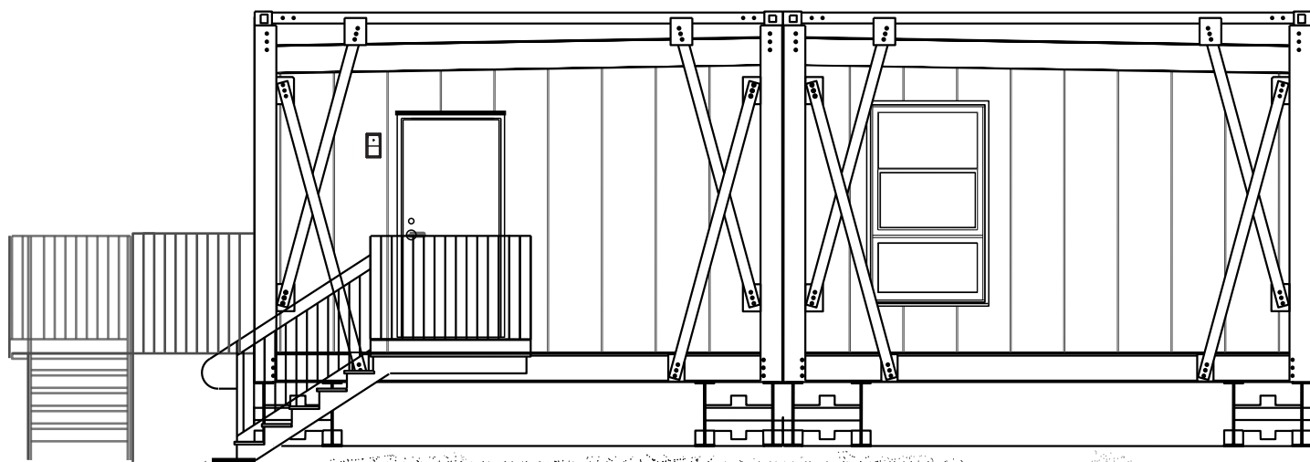
ÉLÉVATION ARRIÈRE
