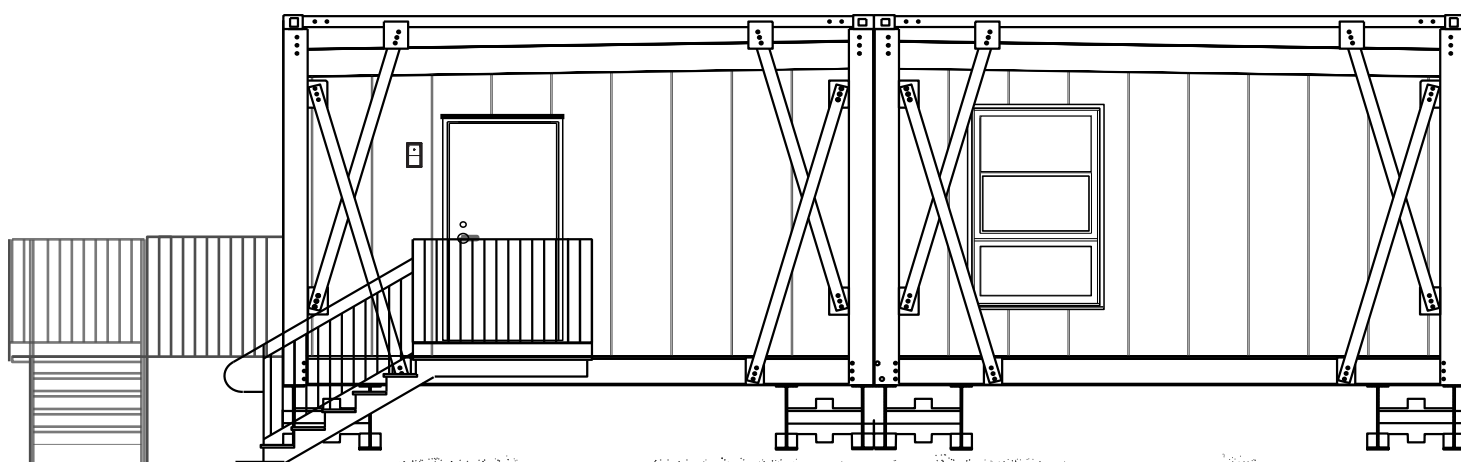
ÉLÉVATION ARRIÈRE
