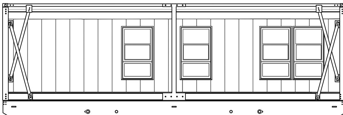
ÉLÉVATION ARRIÈRE
