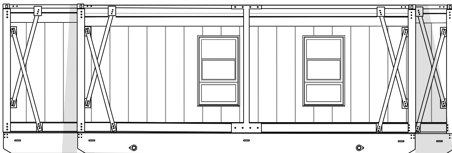
ÉLÉVATION CÔTÉ
