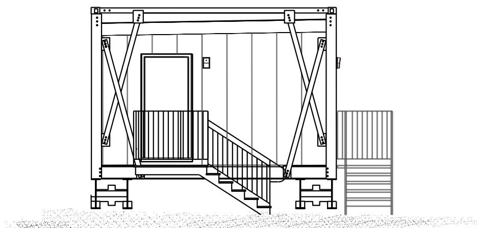
ÉLÉVATION ARRIÈRE
