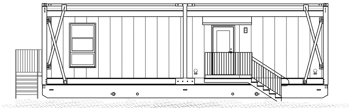
ÉLÉVATION CÔTÉ ENTRÉE
