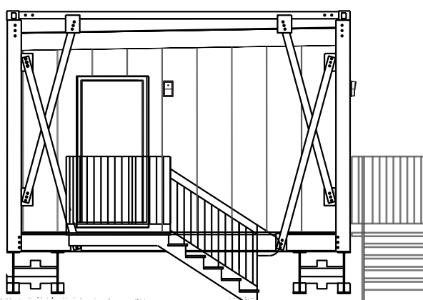
ÉLÉVATION ARRIÈRE
