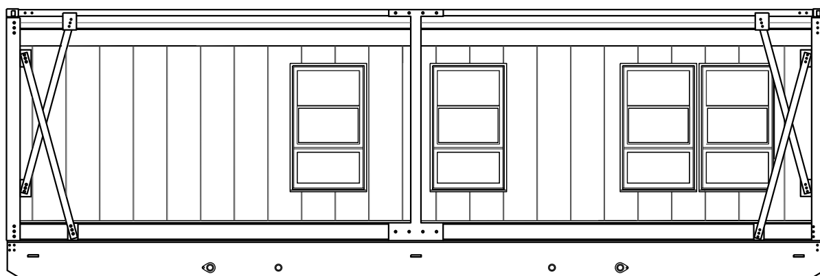
ÉLÉVATION ARRIÈRE
