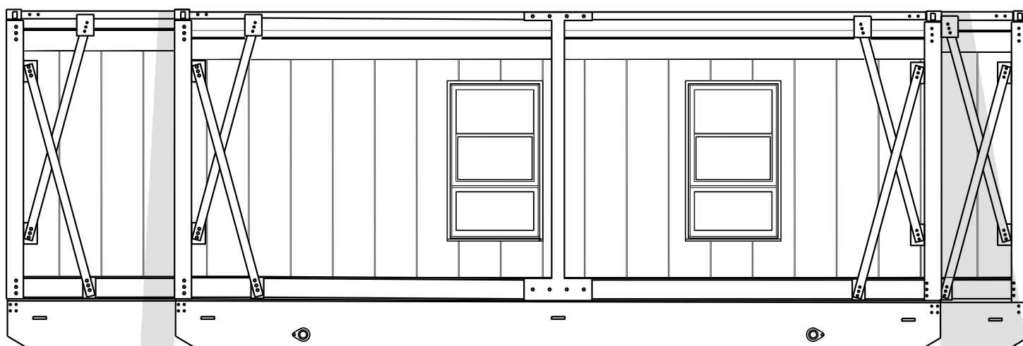
ÉLÉVATION CÔTÉ
