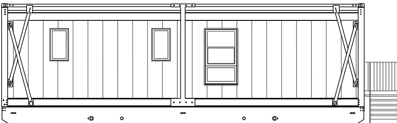
ÉLÉVATION ARRIÈRE
